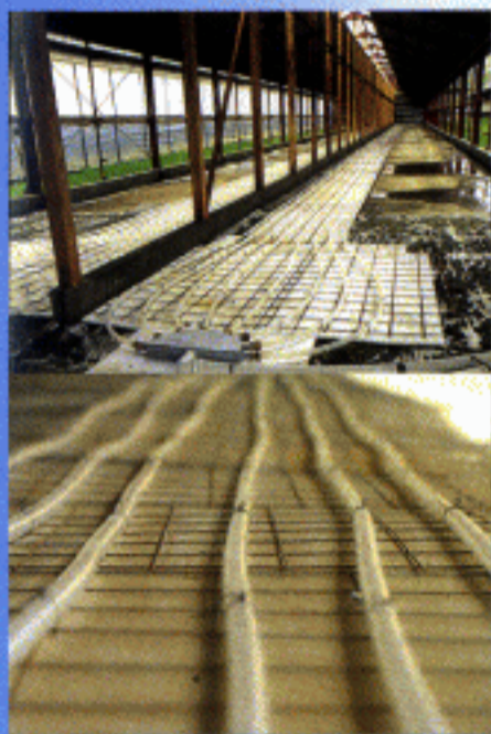
床面暖房システム
